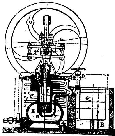
Фиг. 4. Машина съ хлорформнымъ моторомъ Венса (Vincent).
